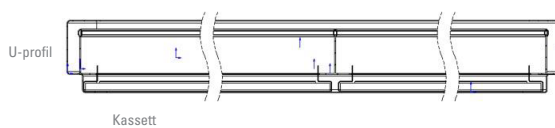
C. Genomskärning – kassetter med avslut S
