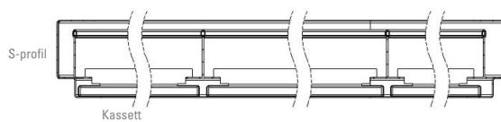
C. Genomskärning – kassetter med avslut S
